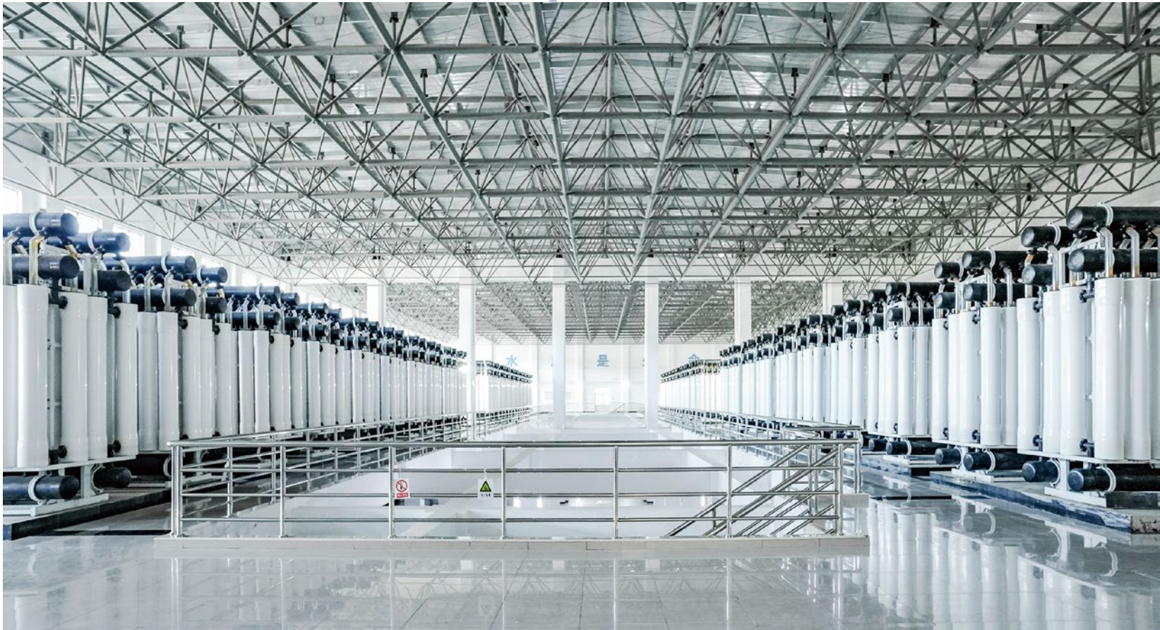
■ 北京南水北调石景山水厂 产水规模：200,000 m 3 /d 核心工艺：BioSecure 生物安全性工艺技术包
